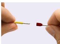
端子により線を挿入する フェールル端子
